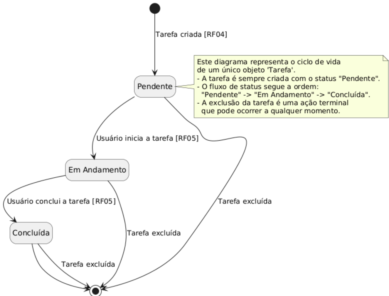
Diagrama de Estado para o Ciclo de Vida de uma Tarefa
